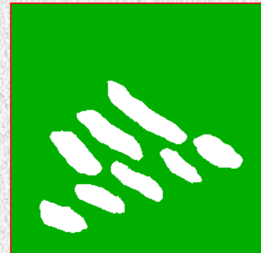
Différence
