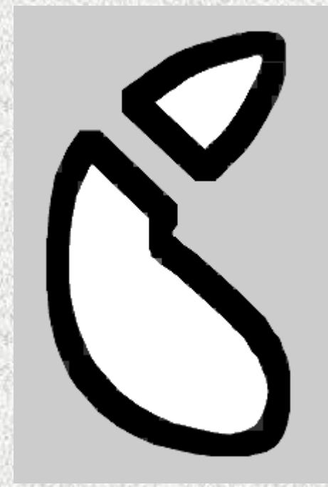
\varepsilon(X^c \cup Y)
